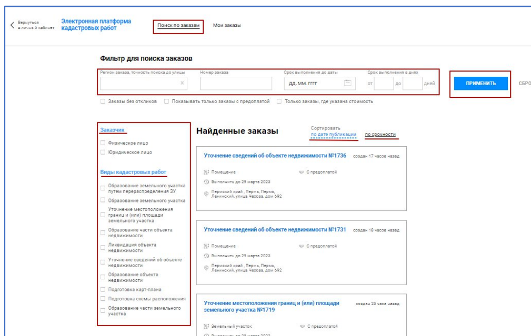
Рисунок 25 – Поиск заказов
