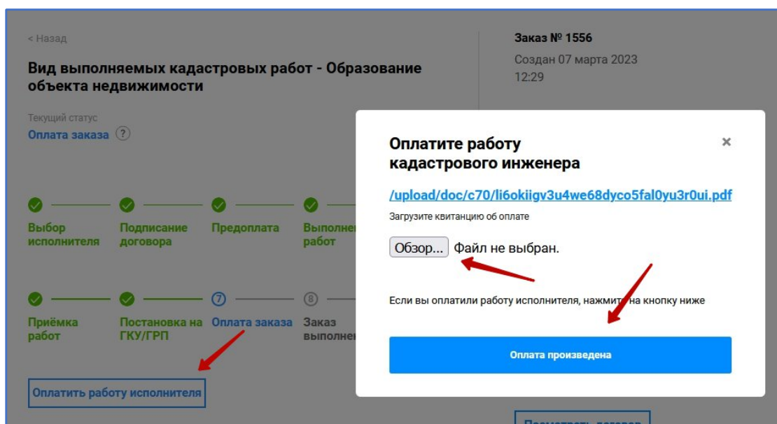
Рисунок 115 – Оплата заказа
