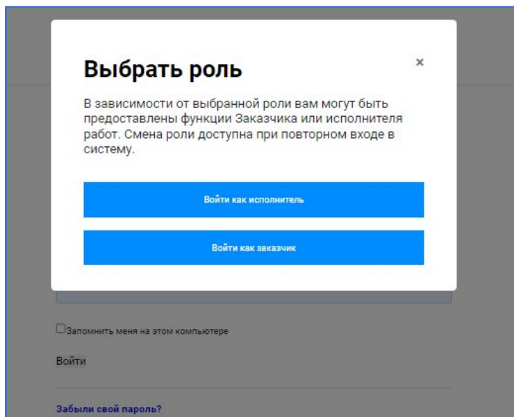
Рисунок 12 – Выбор роли
