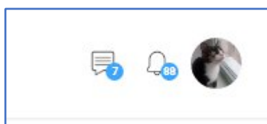
Рисунок 95 – Панель уведомлений
