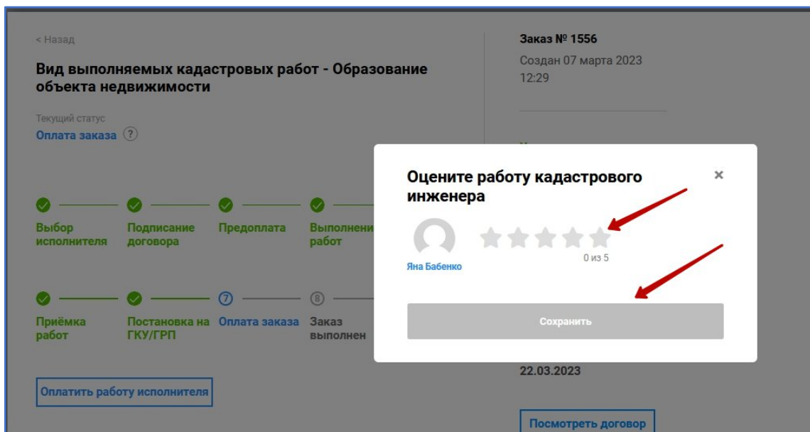
Рисунок 116 – Оценка заказа
