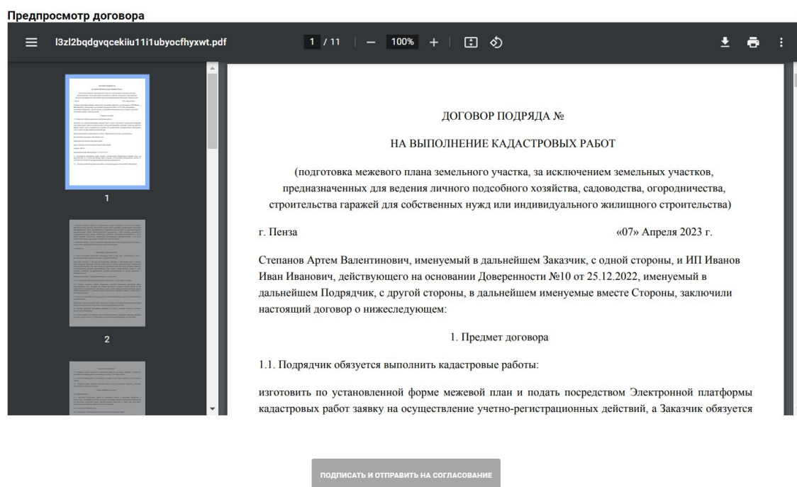
Рисунок 32 – Предпросмотр договора
