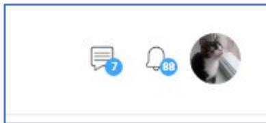
Рисунок 67 – Панель уведомлений
