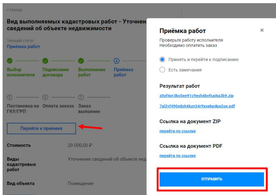
Рисунок 113 – Приемка работ.
