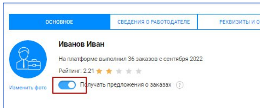
Рисунок 24 – Получение заказов
