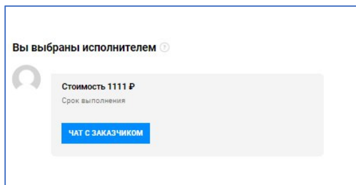
Рисунок 51 – Чат заказа
