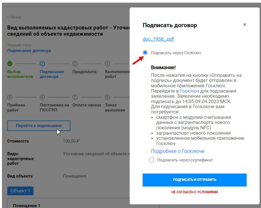
Рисунок 81 – Подписание договора
