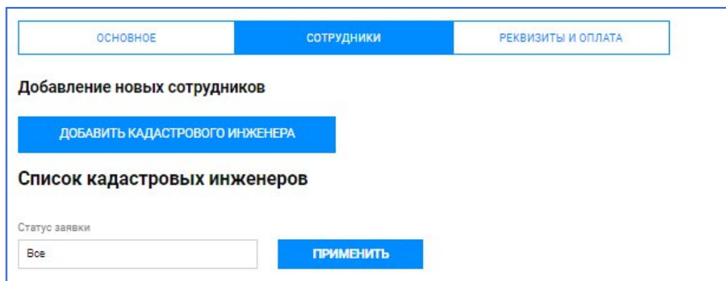
Рисунок 54 – Вкладка «Сотрудники»
