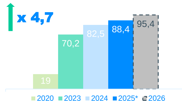
Зоны затопления и подтопления, %
